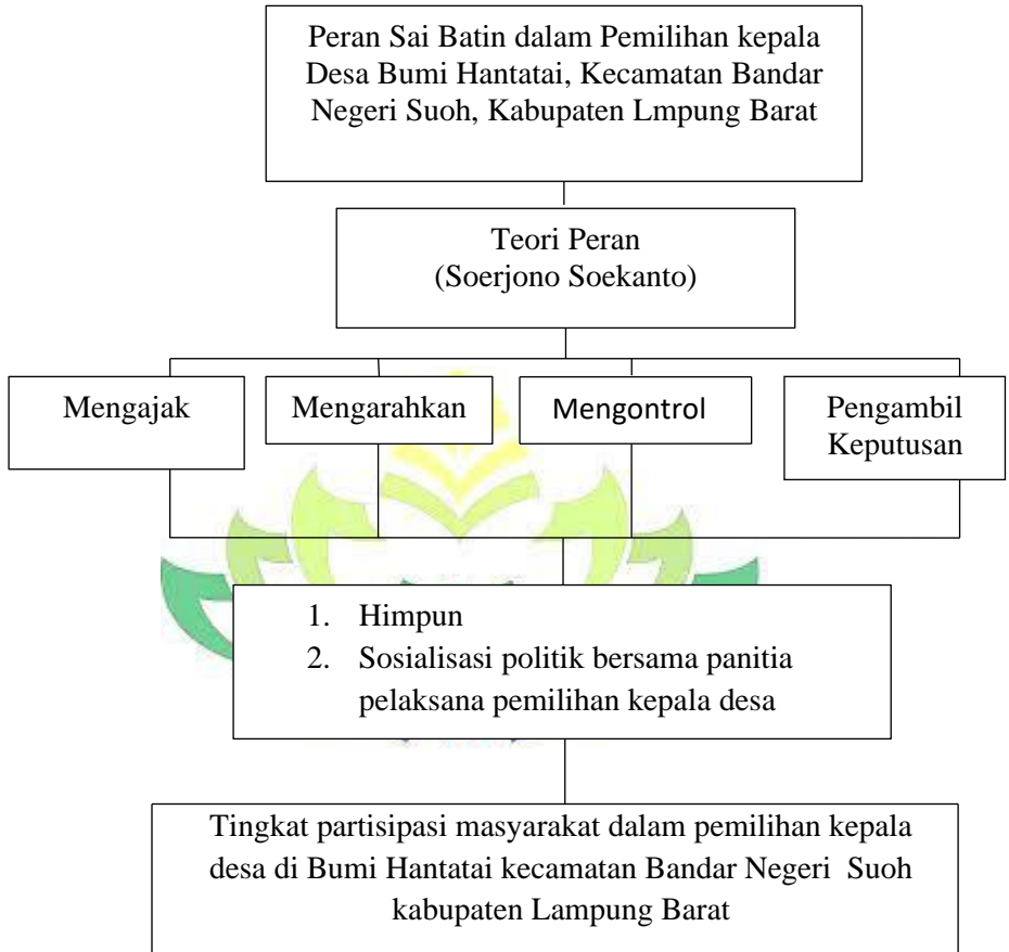
Gambar 1. Kerangka Teori
