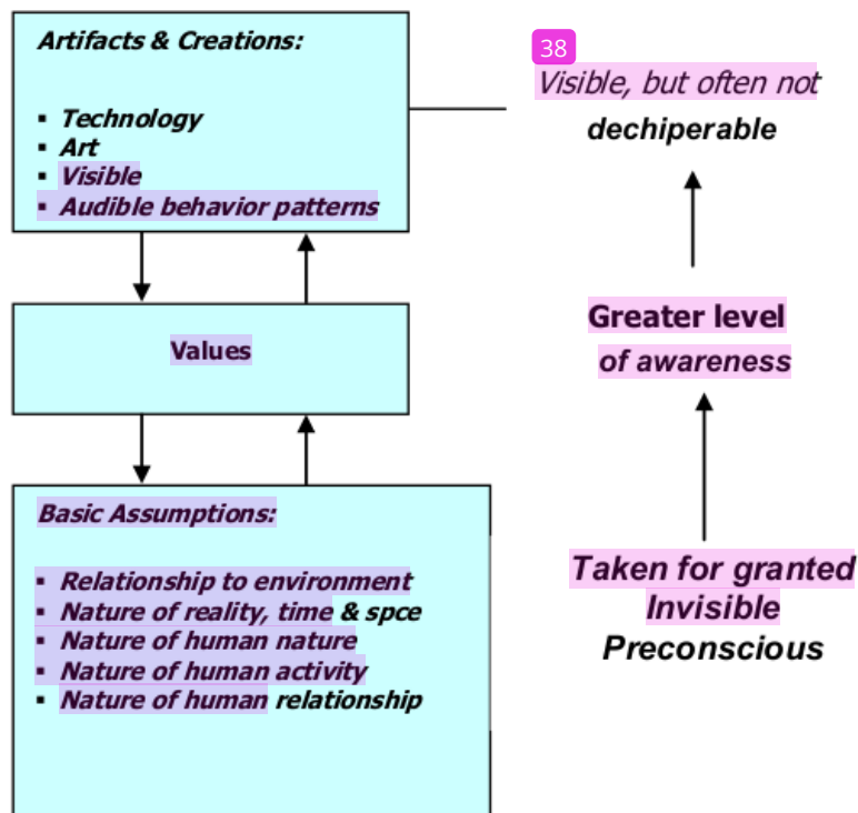
Gambar 7. Jenjang Vudaya
