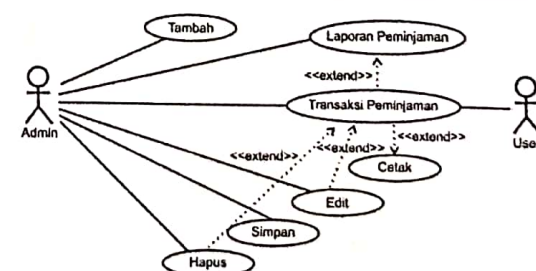
Gambar 5. Use Case Diagram Data Peminjaman
