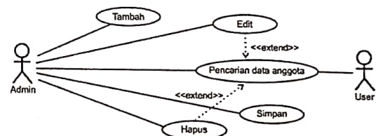
Gambar 3. Use Case Diagram Data Anggota
