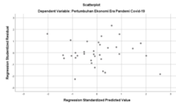
Gambar 1 Uji Heteroskedestisitas
