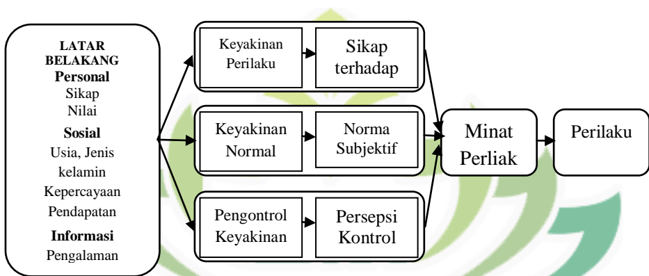
Gambar 1.1 Skema Ruang Lingkup Teori Perilaku Terencana
