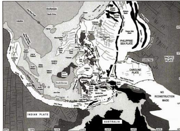
Gambar 1.1 Rekonstruksi lempeng tektonik di Indonesia (Hall, 1995)
